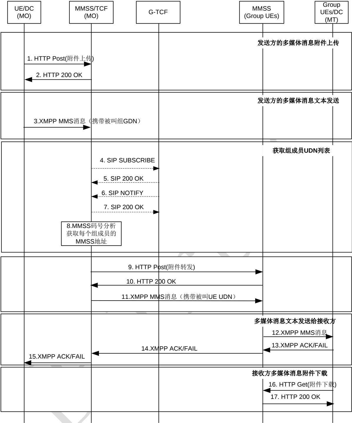
图 17 跨核心网点对群组多媒体消息端到端流程
