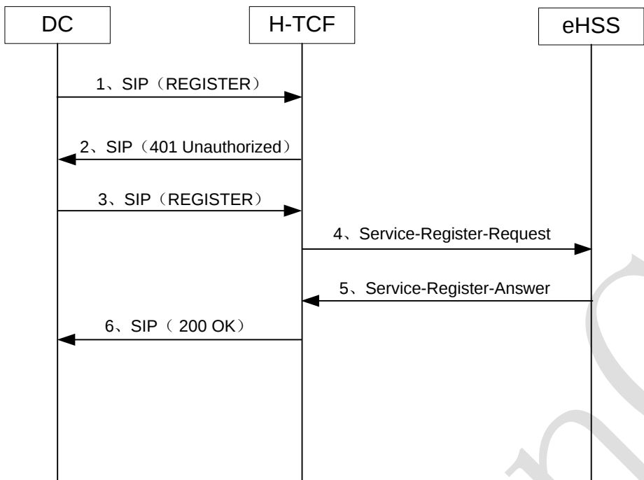
图 21 DC 初始获得 MMSS 地址过程
