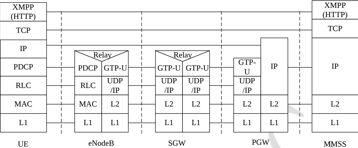
图 3 UE-MMSS 协议栈
