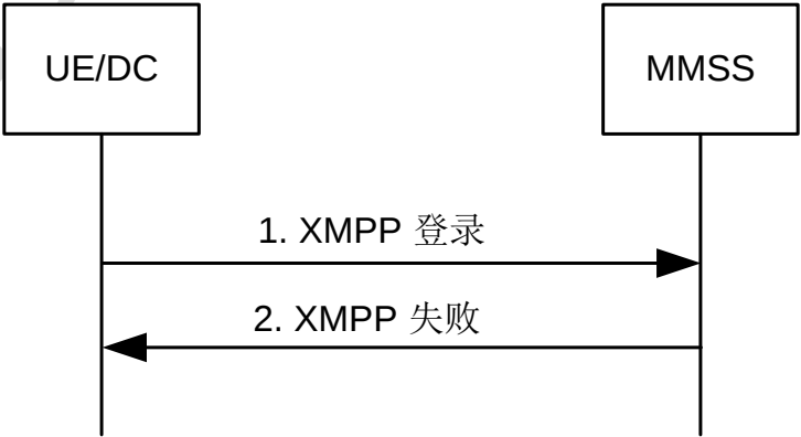
图 9 登录失败流程——用户未签约
